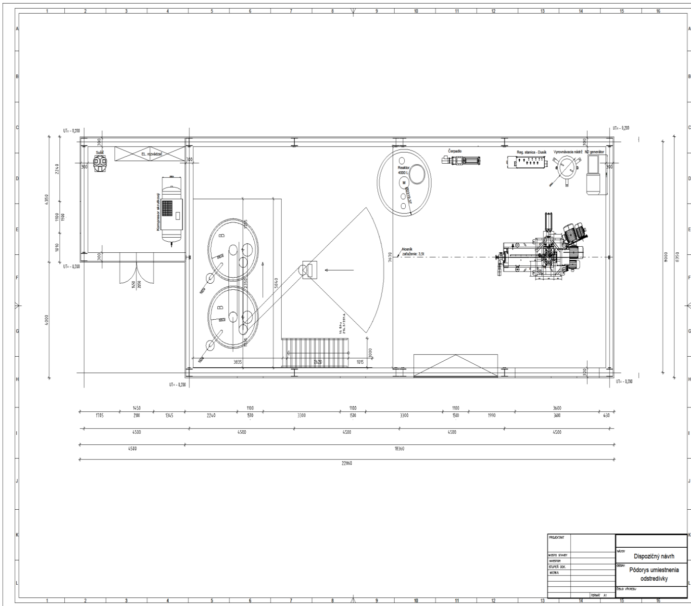
Pôdoris výrobnéj haly CALENDULA a.s
