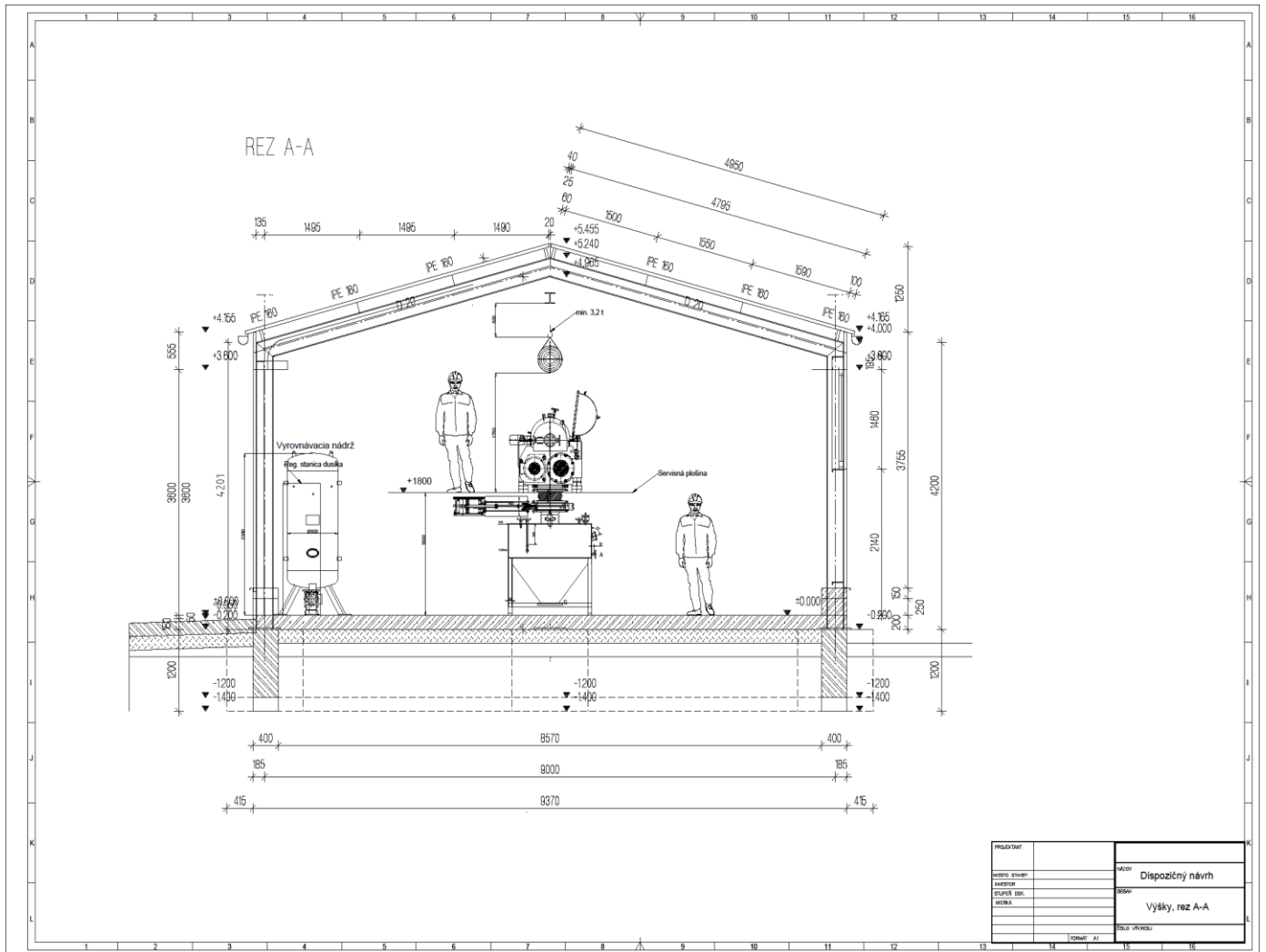
Rez výrobnjej haly
