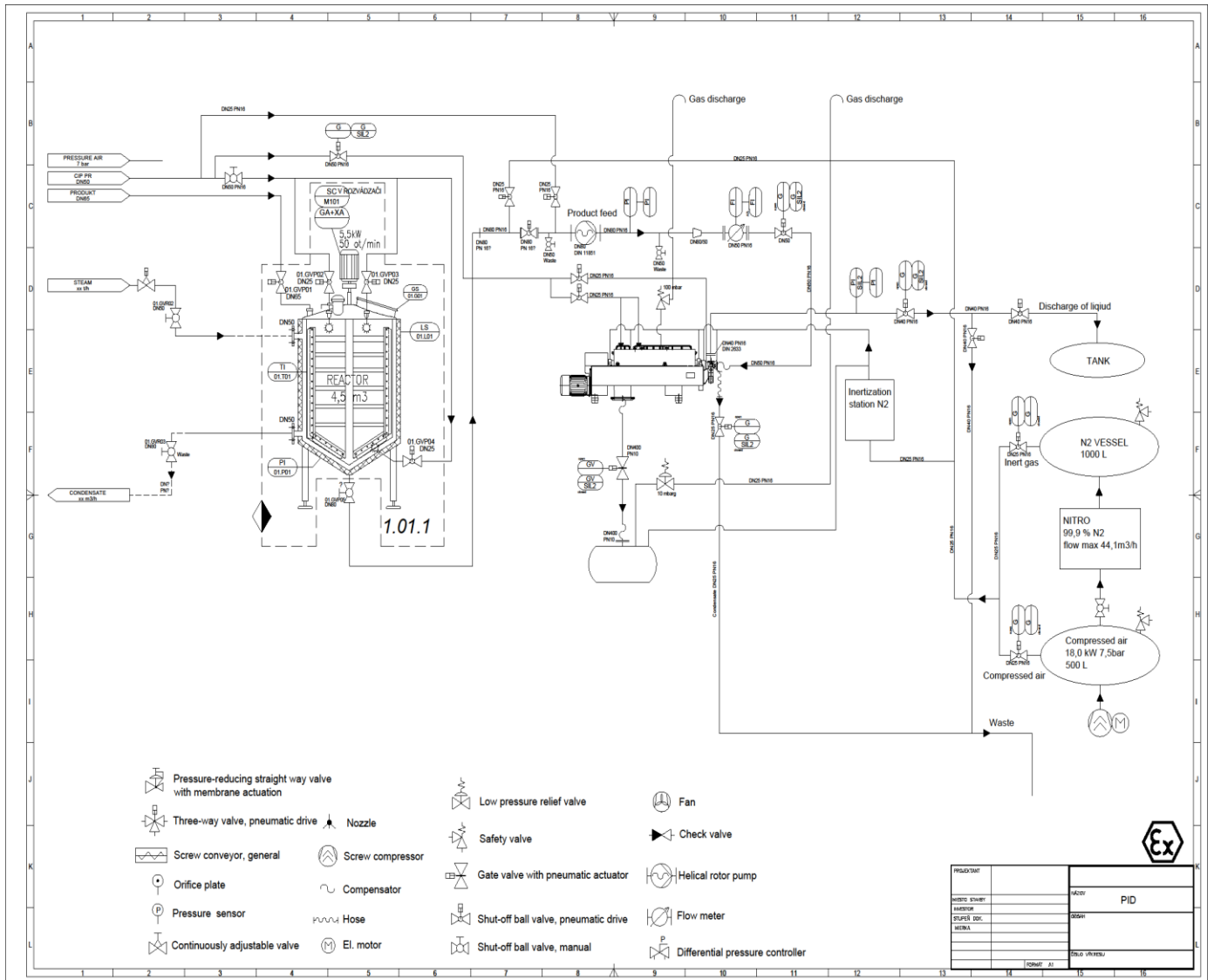
Technická schéma zapojenia linky
